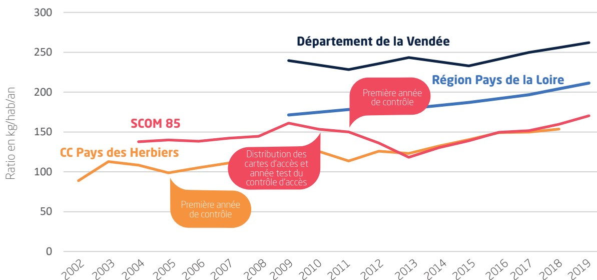
Évolution des ratios des déchets de déchèterie (hors déchets verts) dans la Région Pays de la Loire
